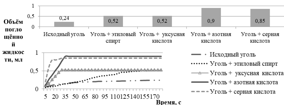
Смачиваемость угольной поверхности водой в модельных системах
